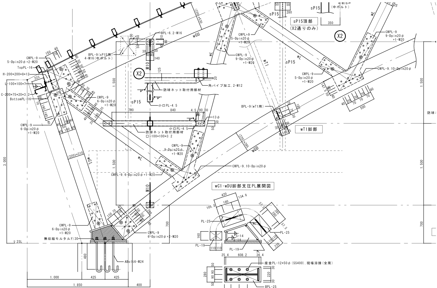
X2通り集成材架構詳細図
